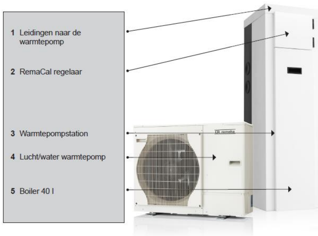
Hybrid Plus 40-5c Hybride binnendeel met warmtepomp.
