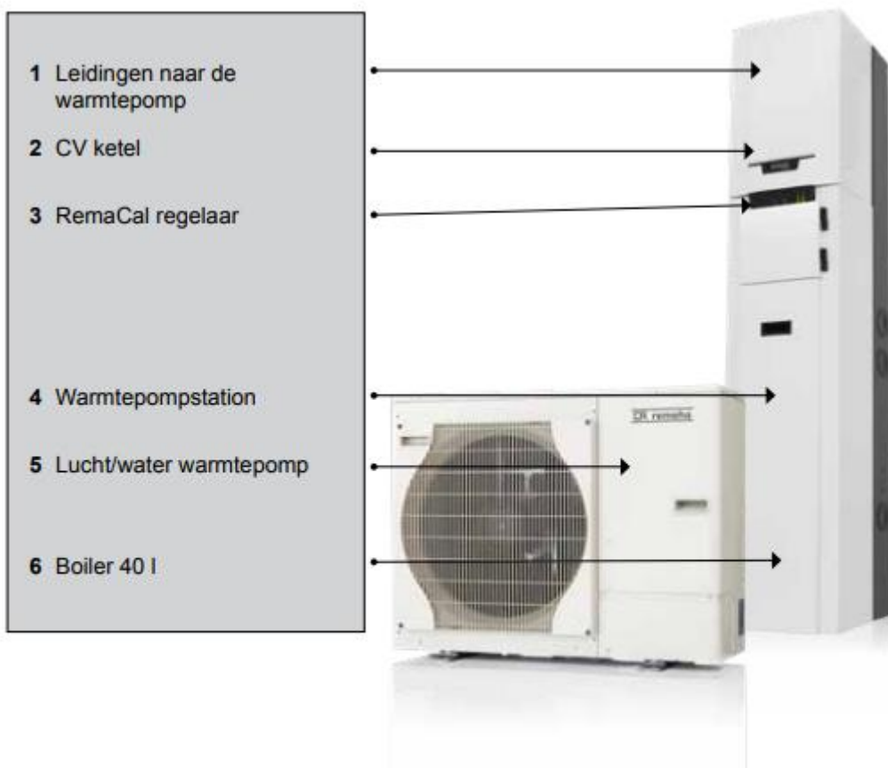
Tzerra HP 40-5c Hybride binnendeel met warmtepomp en CV ketel.
